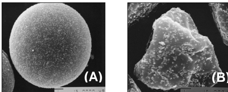
図 重合法トナー(A)と粉砕法トナー(B)の電子顕微鏡写真
