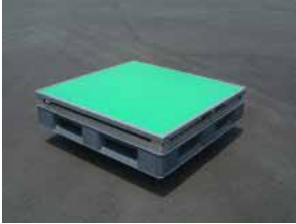
「ステックNL型Sタイプ」の折りたたみ状態 (組み立て状態の高さの 1/4 の高さ)
