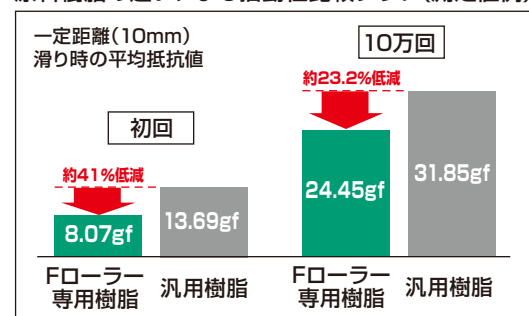
原料樹脂の違いによる摺動性比較グラフ（測定値例）
