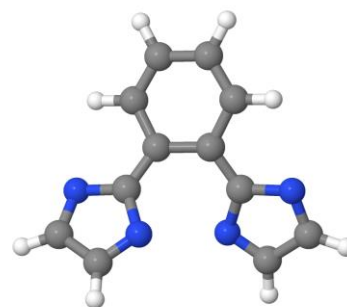
図 1. 計算したモノアリルジイミダゾールの構造。グレーは炭素、白は水素、青は窒素を表します。
