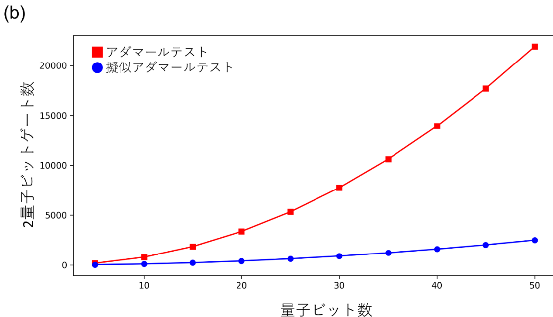
図 3. 疑似アダマールテストの概要とリソース比較
