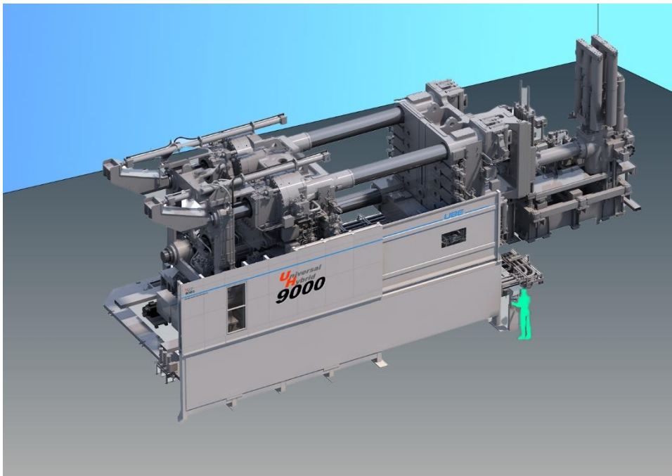
UH9000 ダイカストマシンの外観（イメージ図）
